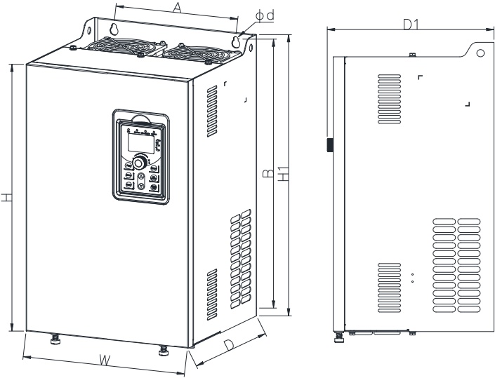
图 4-11： 30~220kW G3 外形尺寸（机座号：A5~A11，A19）
