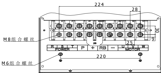
图 4-24: 75kW G3B 主回路端子 (机座号: A19)
