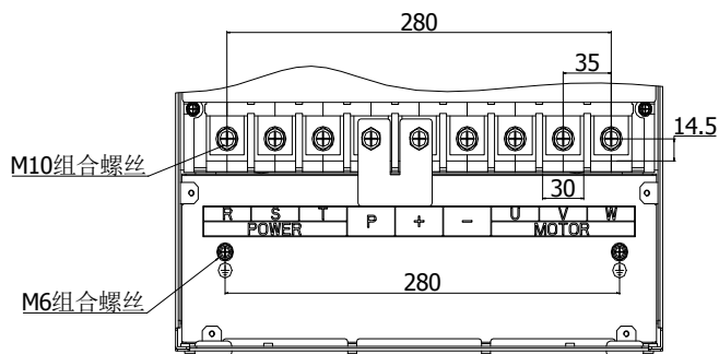
图 4-26: 93~132kW G3/F3 主回路端子图 (机座号: A9)
