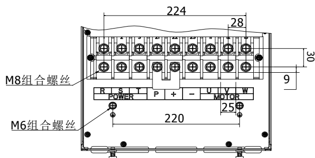
图 4-25: 75kW G3/F3 主回路端子图 (机座号: A8)
