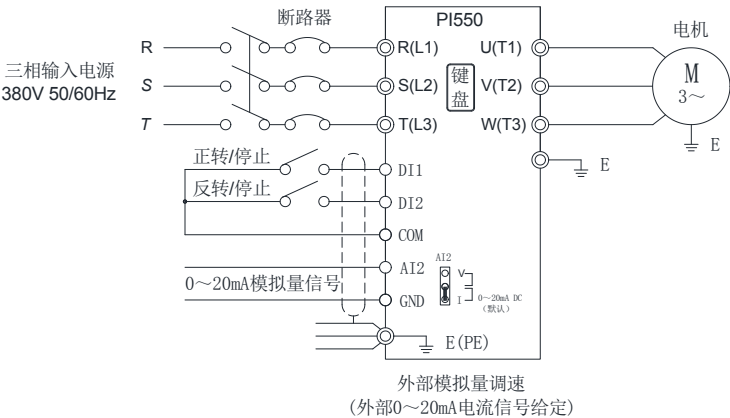
7-13-1 电气图：
