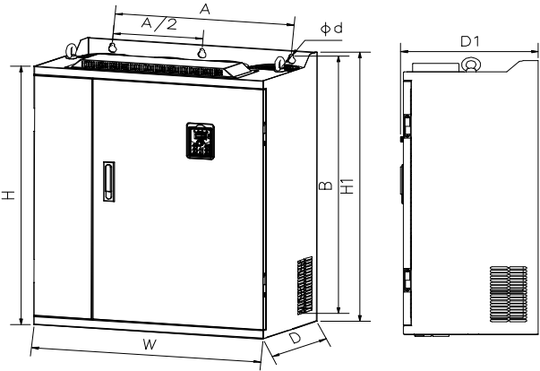
图 4-11： 30~220kW G3 外形尺寸（机座号：A5~A11，A19）
