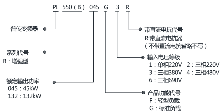
图 3-4 型号说明
