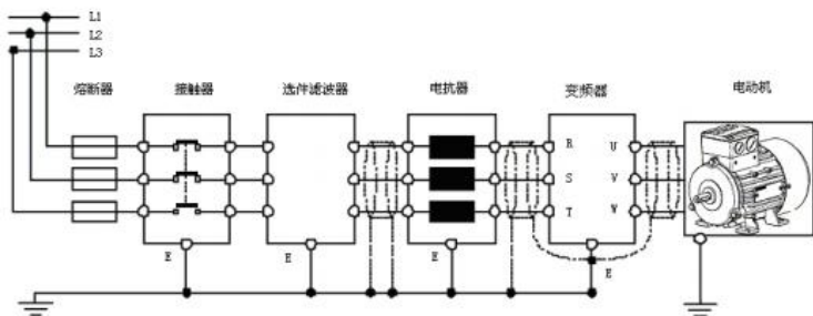
图 4-2： PI550 系列变频器系统接地图
