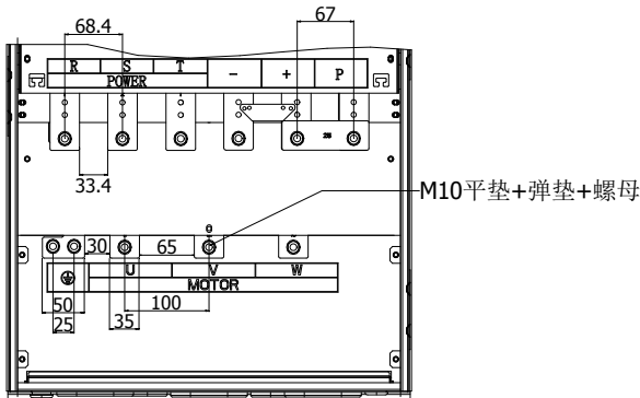
图 4-28： 187~220kW G3/F3 主回路端子（机座号：A11）
