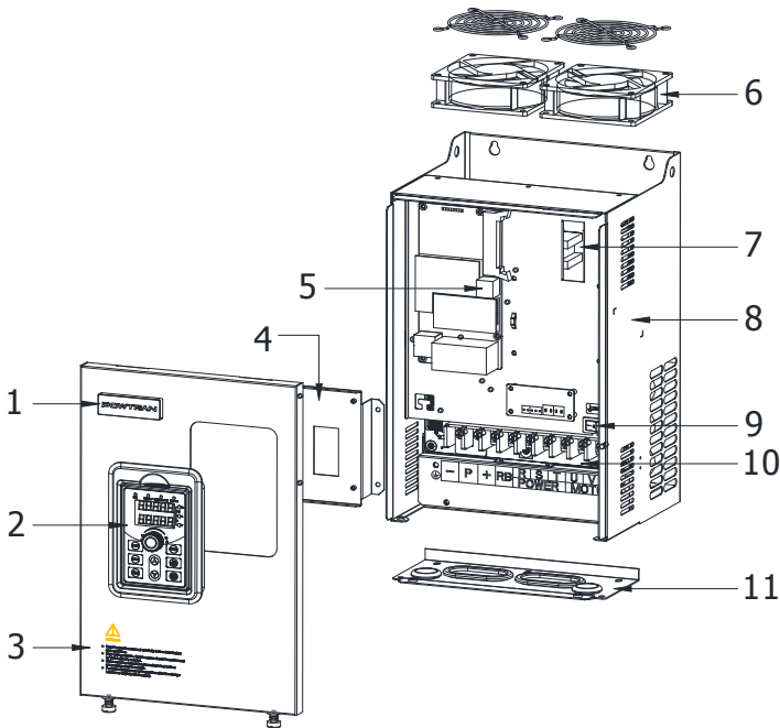
图 4-4：铁壳机结构示意图
