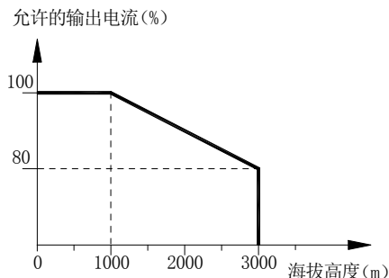
图 2-2: PI550 系列变频器超海拔降额曲线图
