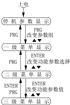
图 5-2：操作流程图
