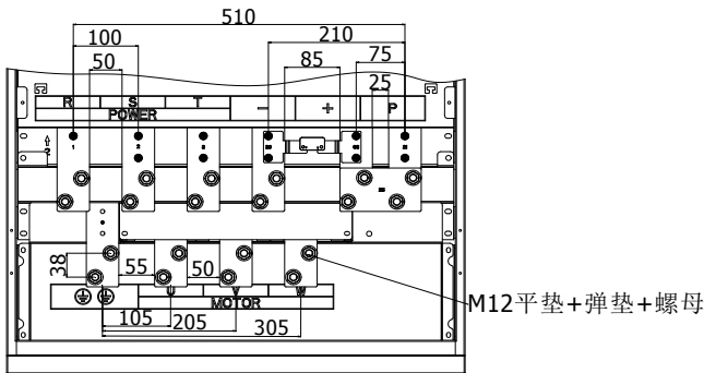
图 4-29： 250~450kW G3/F3 主回路端子（机座号：A12~A13）
