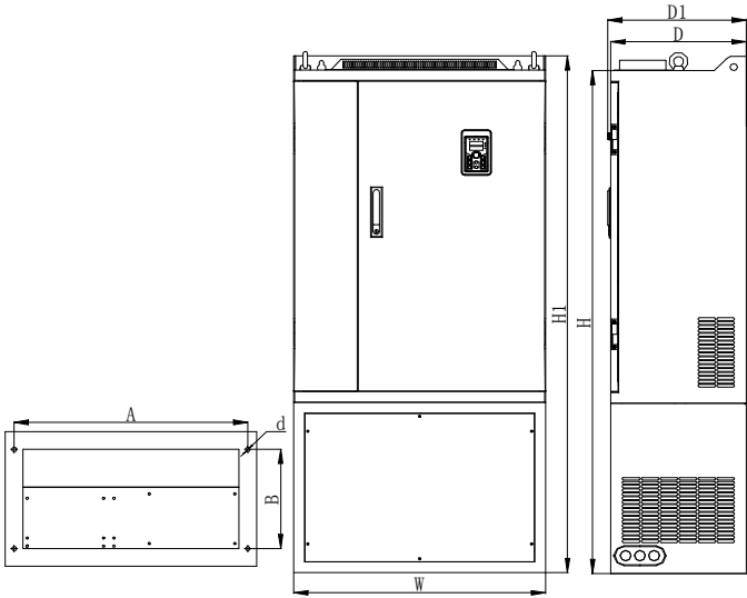
图 4-13： 132~220kW G3R （机座号：A13.1, A14~A15）
