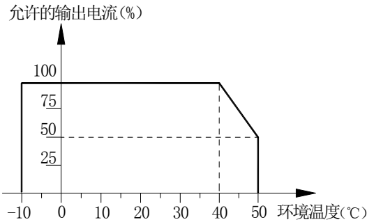
图 2-1: PI550 系列变频器超温降额曲线图
