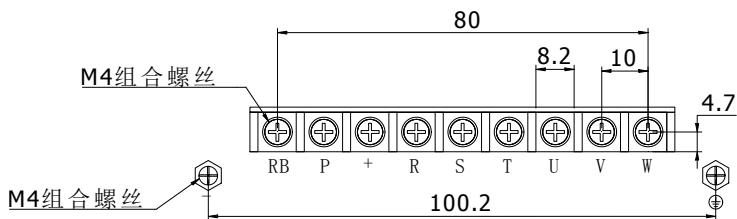
图 4-19： 5.5~11kW G3 主回路端子图（机座号：A3）
