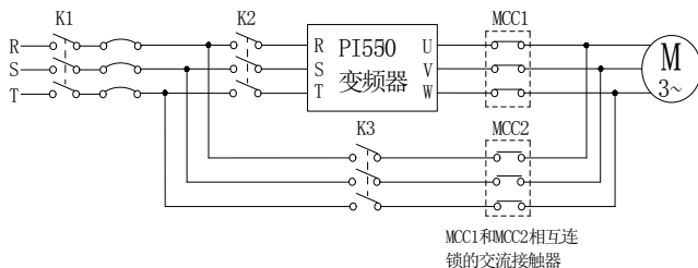
图 4-40：备用电路电气图
