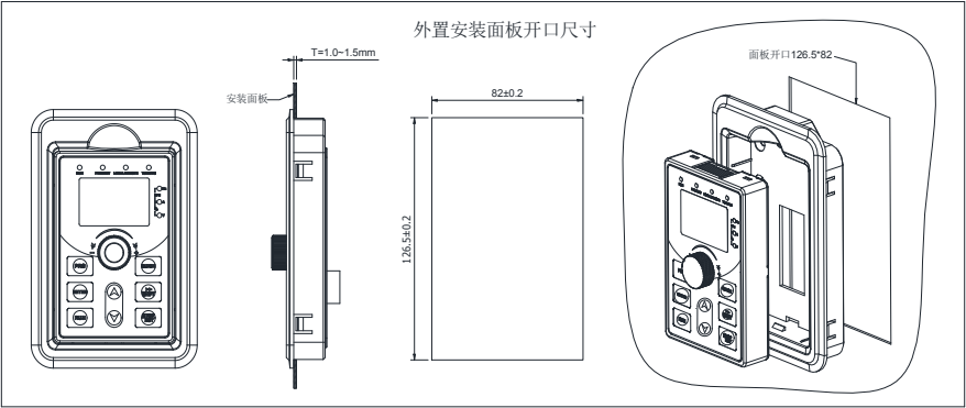
图 4-17： 键盘安装开口尺寸图(尺寸单位：mm)
