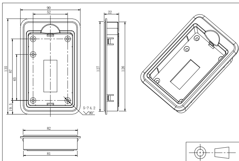
图 4-16: 键盘仓尺寸图(尺寸单位: mm)
