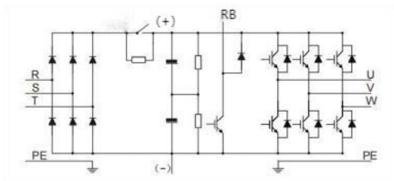
图 3-1 0.7~4kW 主回路简图
