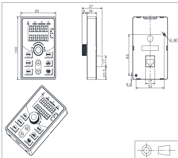
图 4-15: PI550 键盘尺寸图(尺寸单位: mm)
