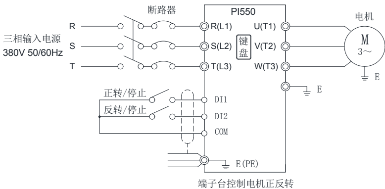
7-5-1 电气图：
