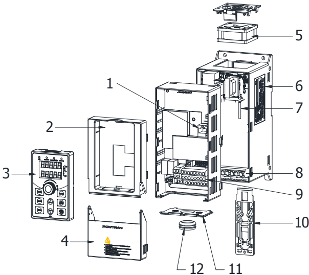
图 4-3： 塑壳机结构示意图
