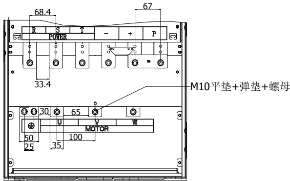
图 4-27： 160kW G3/F3 主回路端子（机座号：A10）
