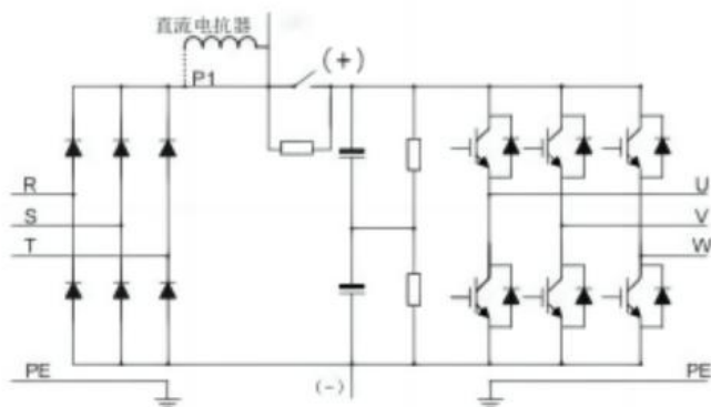
图 3-2 37kW 及以上主回路简图
