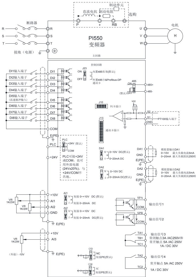
图 4-35：配线图
