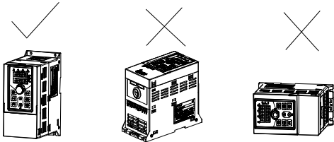
图 4-5： 变频器安装示意图
