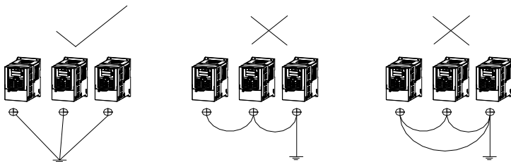
图 4-1： PI550 系列变频器多台并联接地图
