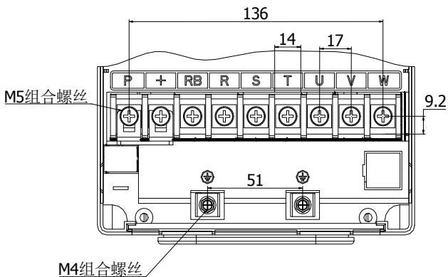
图 4-20： 15~22kW G3/F3 主回路端子图（机座号：A4）
