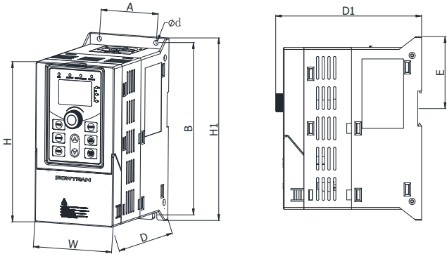
图 4-8： 0.4~4kW G3 外形尺寸（机座号：A1~A2）
